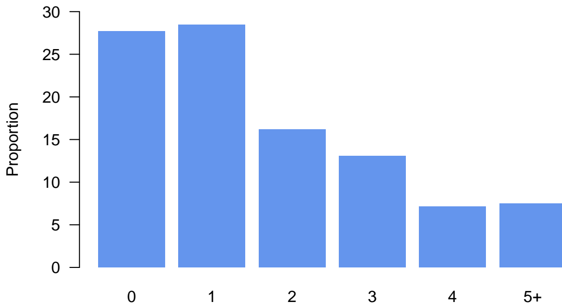
FIGURE 3 – Diagramme en barres pour la variable Nombre d'enfants
