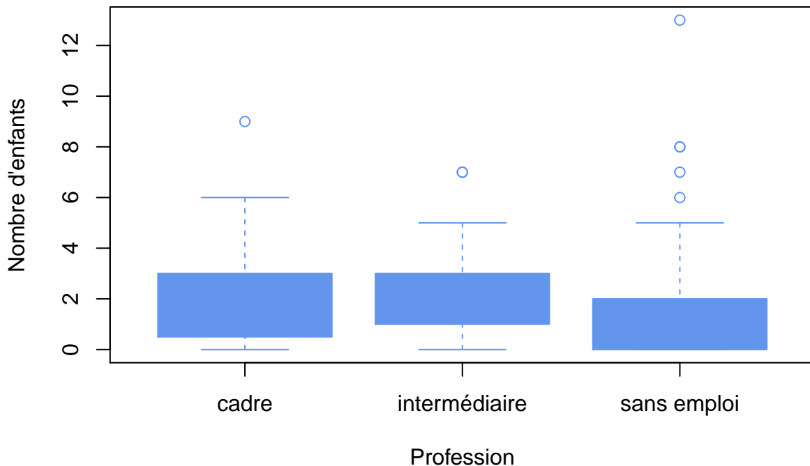
FIGURE 10 – Diagrammes de type boîte à moustaches (bis)
