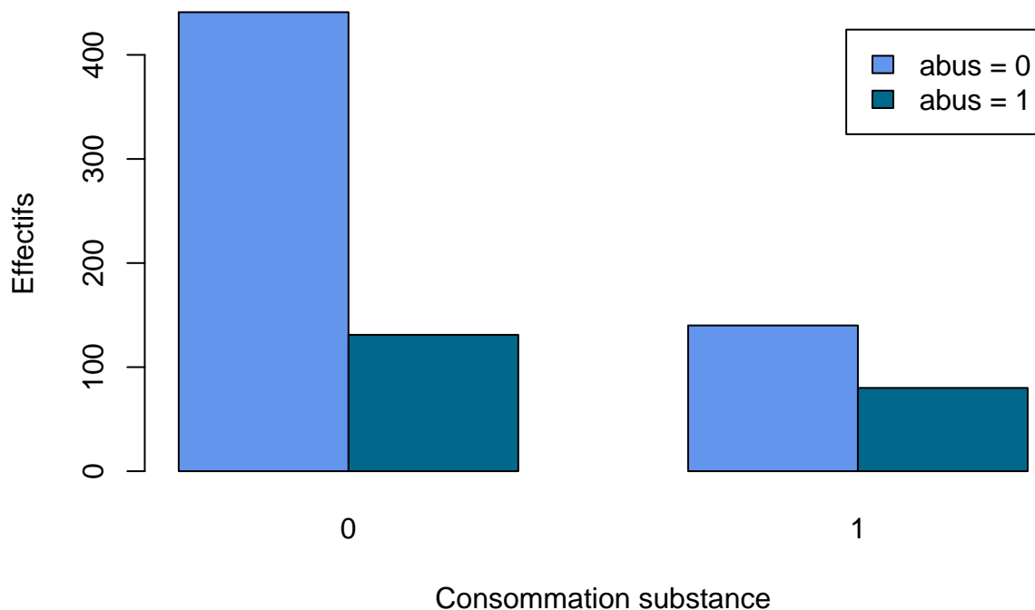
FIGURE 5 – Diagramme en barres pour deux variables qualitatives
