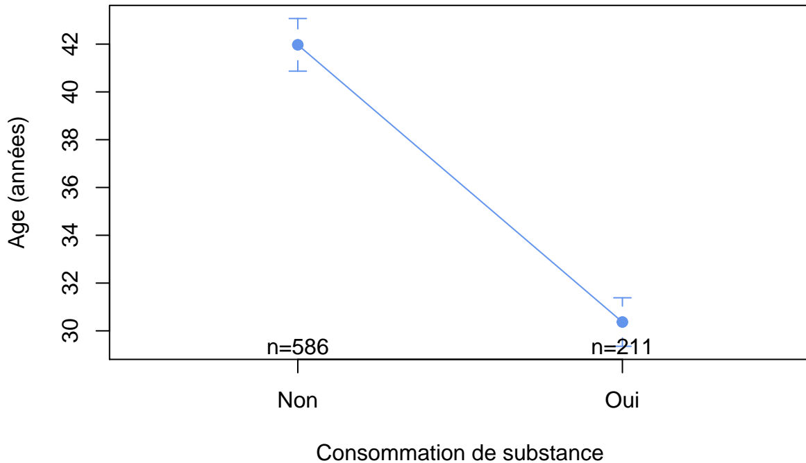
FIGURE 8 – Utilisation de commandes graphiques intégrées du package gplots
