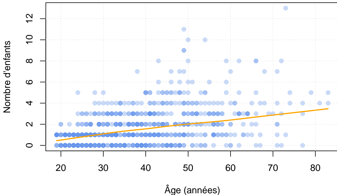
FIGURE 9 – Utilisation de commandes graphiques intégrées du package gplots (bis)
