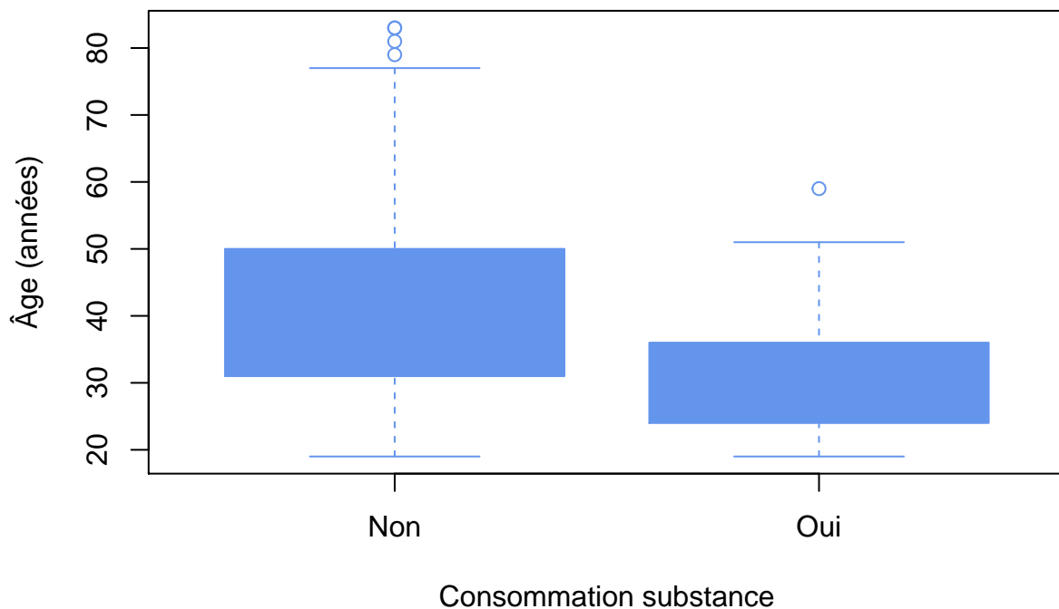
FIGURE 7 – Diagrammes de type boîtes à moustaches
