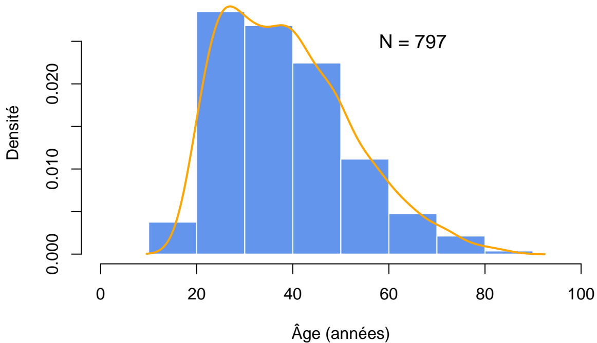
FIGURE 4 – Histogramme (densité) pour la variable Age
